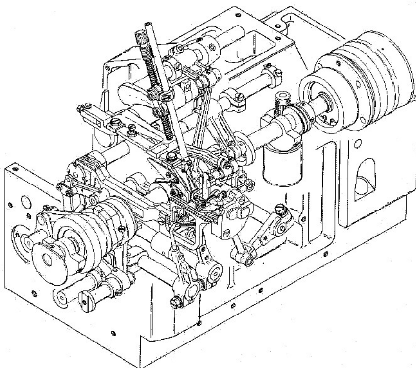
PERSPECTIVE 透視図
