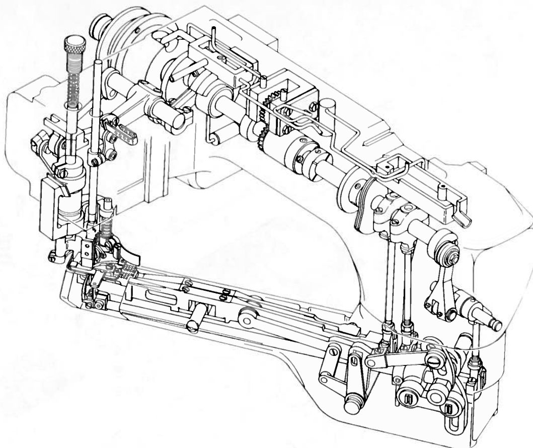
PERSPECTIVE 透視図
