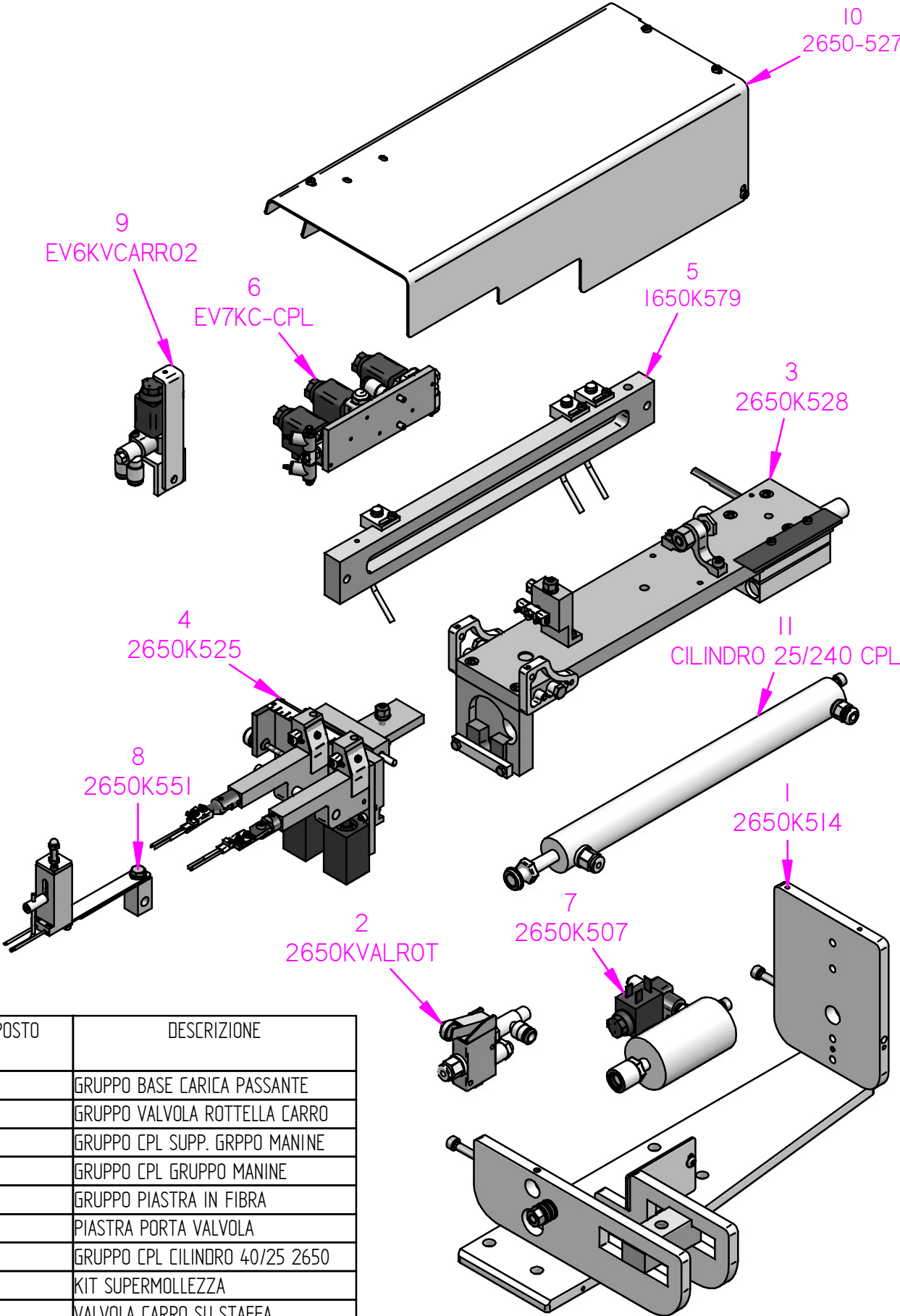
3650KCARRO APPARECCHIATURA COMPLETA CARICAMENTO PASSANTI
