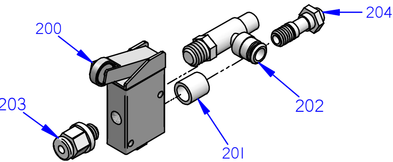
2650KVALROT GRUPPO VALVOLA A ROTTELLA CARRO
