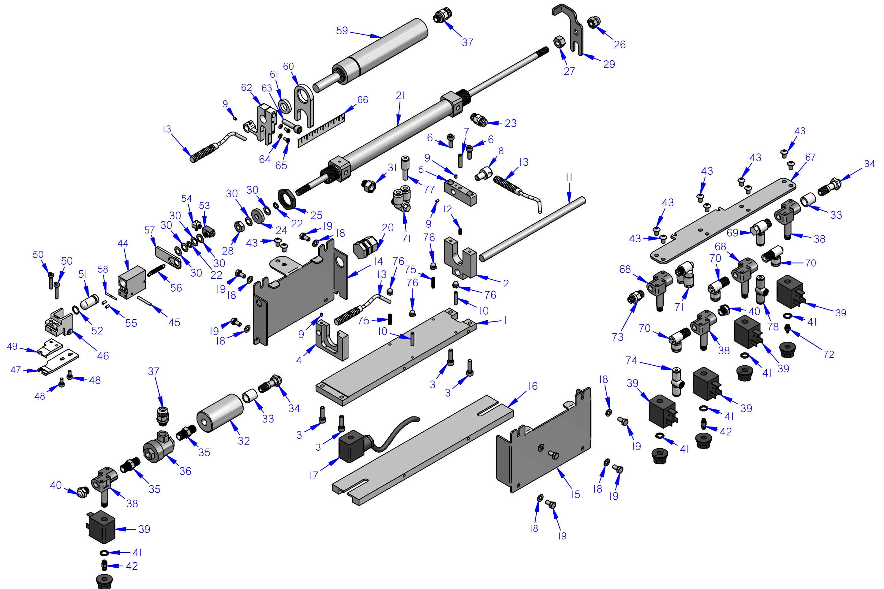
TAVOLA 7 DISPOSITIVO TIRAPASSANTE TABLE 7 LOOP PULLING ASS.
