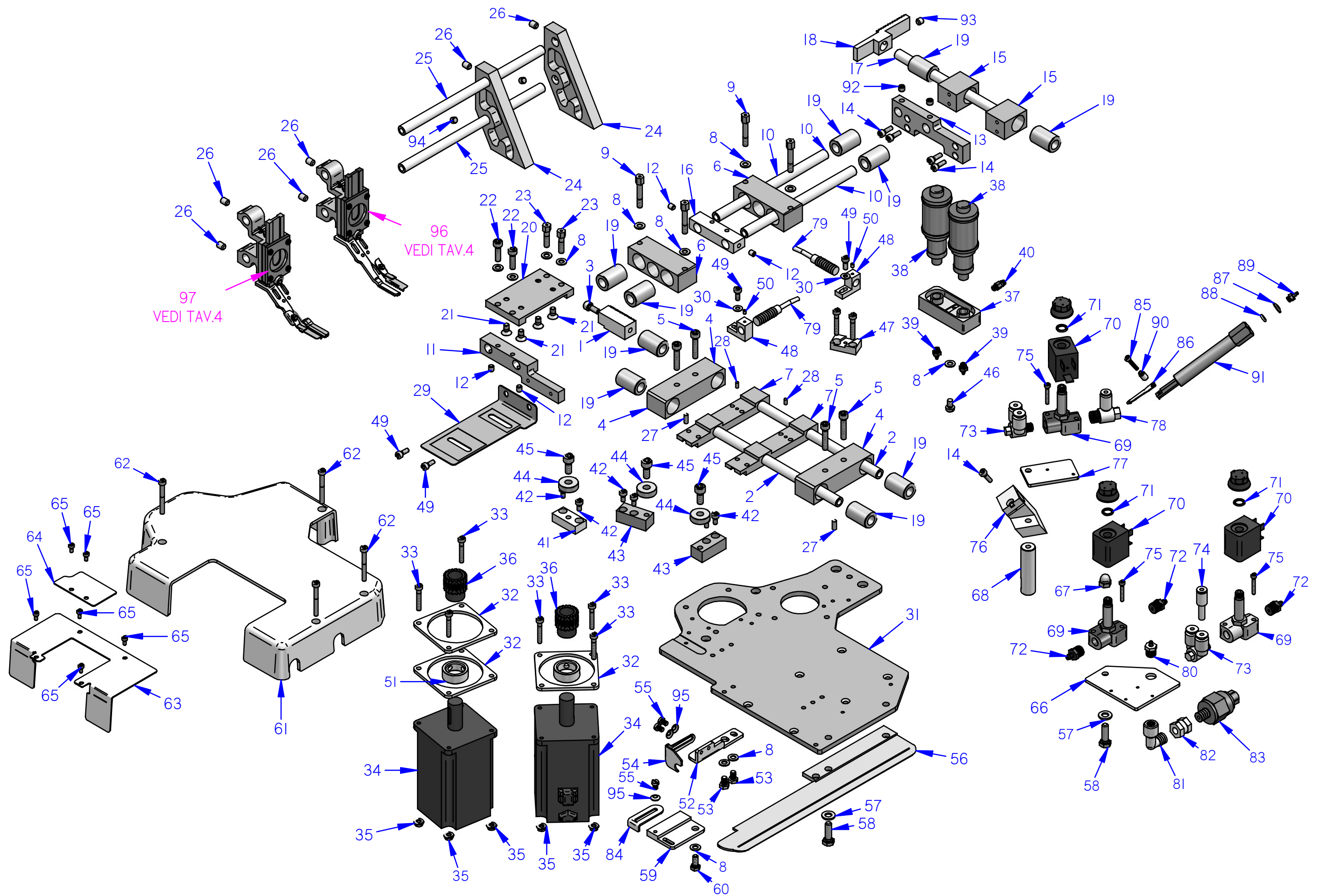
TAVOLA 3 MECCANISMI TRASPORTO TESSUTO TABLE 3 SEWING FEEDING MECHANISM
