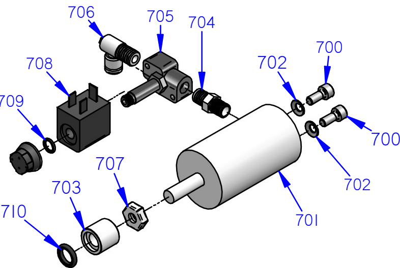
2650K507 GRUPPO COMPLETO CILINDRO 40/25 2650
