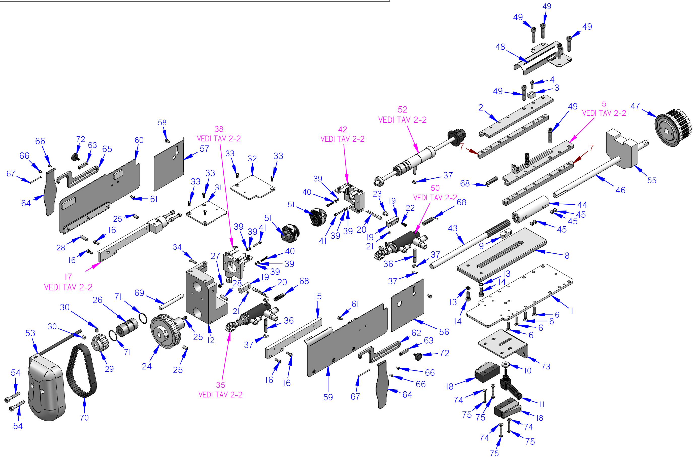
TAVOLA 2-1 TESTA CUCITRICE
