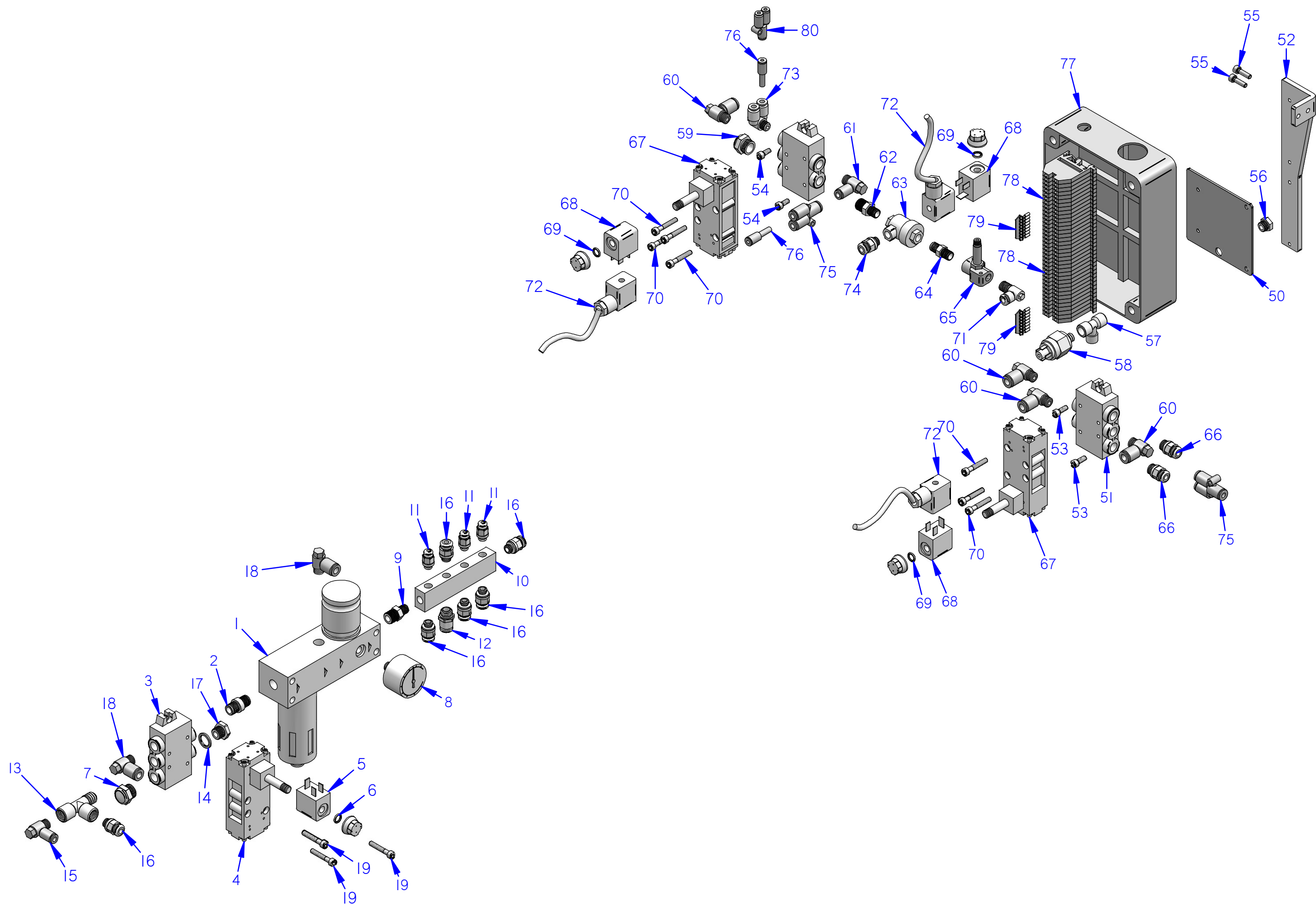
TAVOLA 10 GRUPPO ARIA E GRUPPO VALVOLE TABLE 10 AIR AND VALVES ASS.
