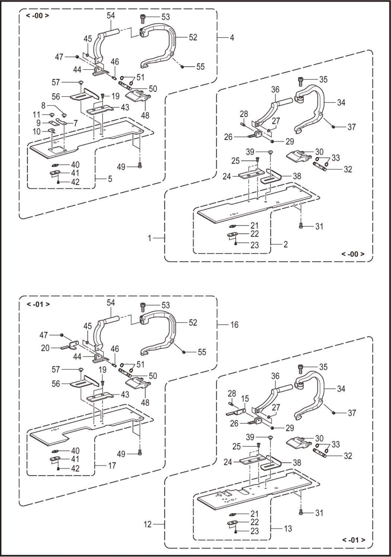
F2 . 压脚装置 / Presser foot mechanism
