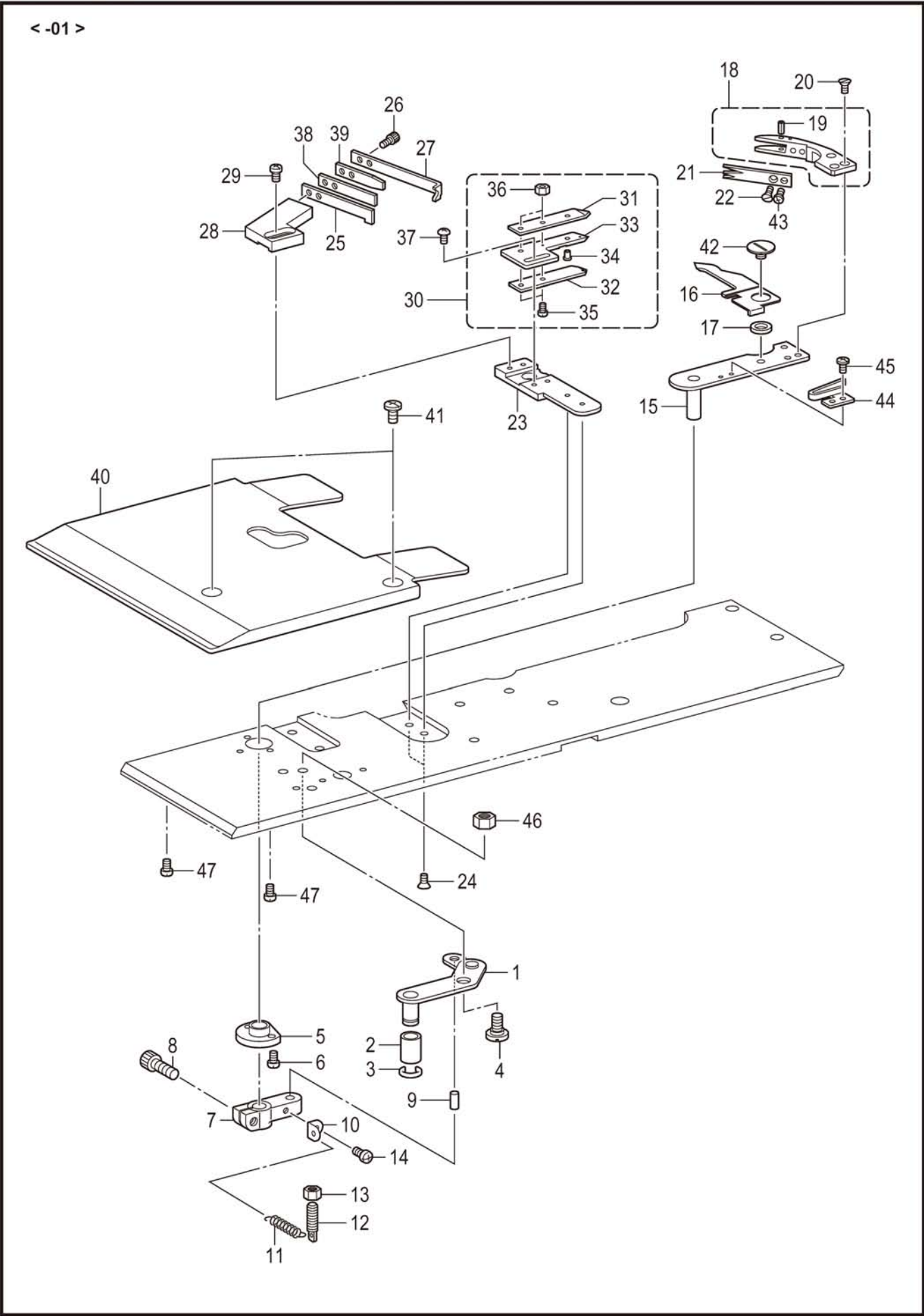
Q1. 切线装置 / Thread trimmer mechanism
