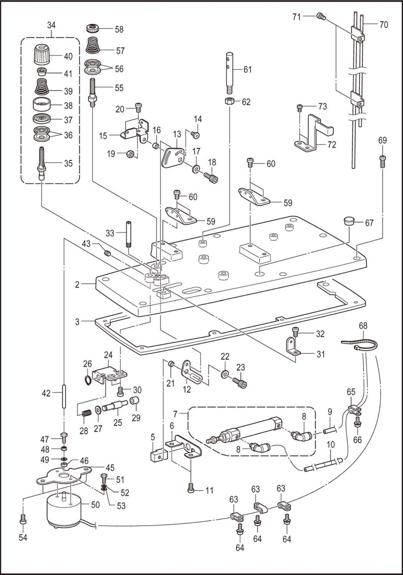
P1. 穿线装置 / Threading mechanism
