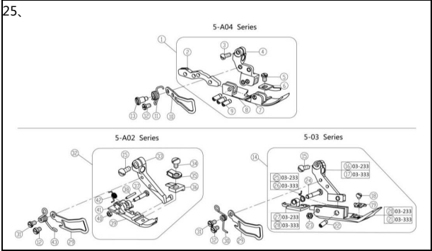
二十五、专用零件/Specific Parts
