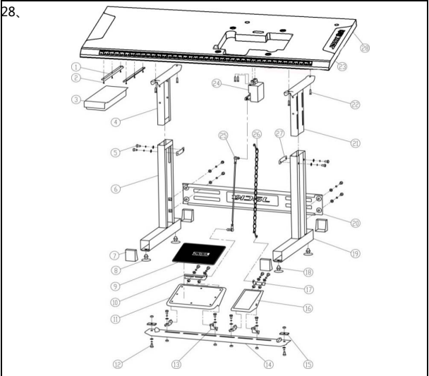
二十八、机架部件/machine stand table assy
