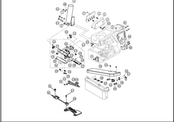
二十六、专用零件/Specific Parts
