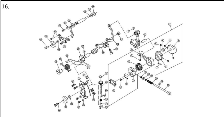
十六、差动调节机构/Feed Mechanism
