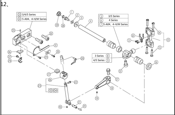
十二、上弯针部件/Upper Loper Drive Mechanism
