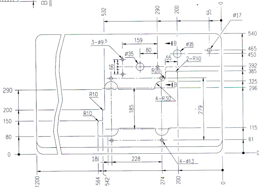
三針筒車下乘式桌板圖 C007/C858 SERIES TABLE CUT-OUT SEMI-SUBMERGED FOR 自動切線 單位/UNIT:MM 所有尺寸公差/DIFFERENCE±2
