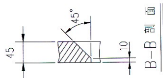
三針筒車下乘式桌板圖 C007/C858 SERIES TABLE CUT-OUT SEMI-SUBMERGED FOR 自動切線 單位/UNIT:MM 所有尺寸公差/DIFFERENCE±2
