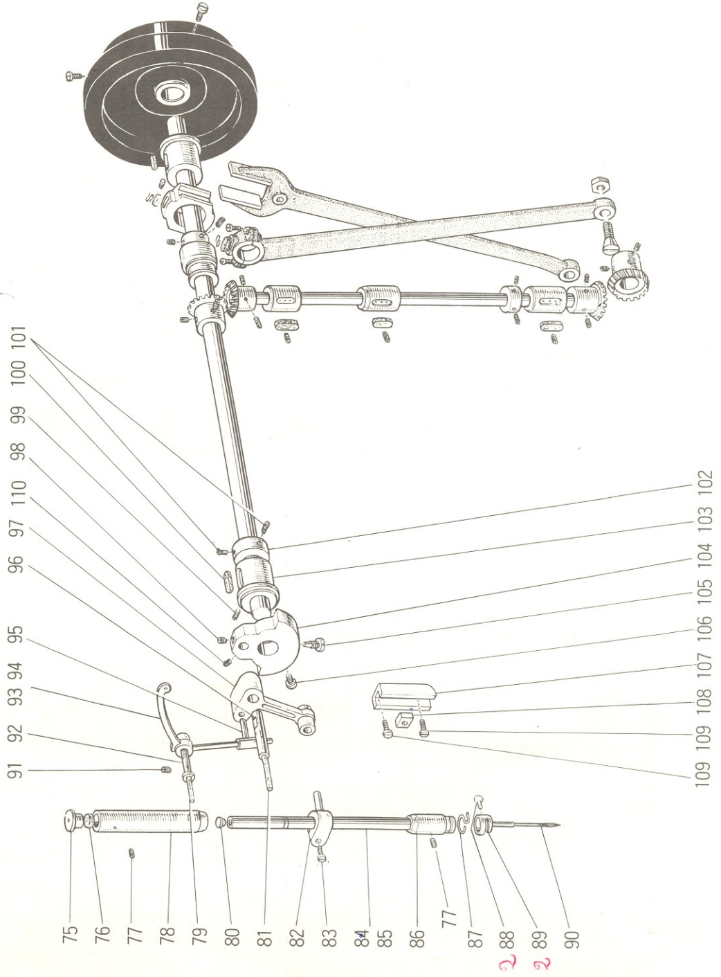
PB-810-10・820-10(PB-810・820)形 針棒、天びん部分 NEEDLE BAR AND TAKE-UP LEVER MECHANISM
