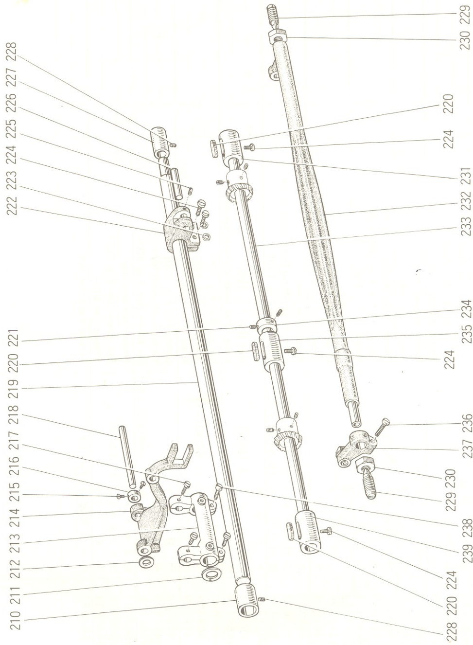
PB-810-10・820-10(PB-810・820)形 下軸, 上下送り軸部分 ROTATING HOOK SHAFT AND FEED LIFTING ROCK SHAFT MECHANISM
