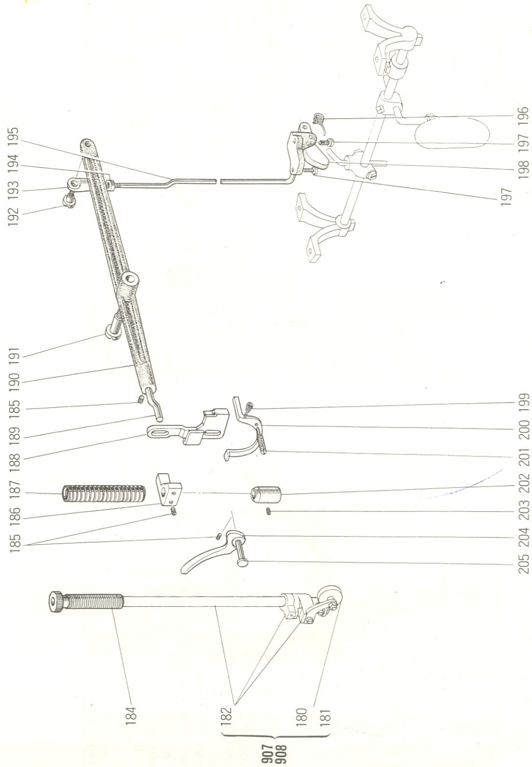
PB-810-10・820-10(PB-810・820)形 押え機構部分 PRESSER FOOT MECHANISM
