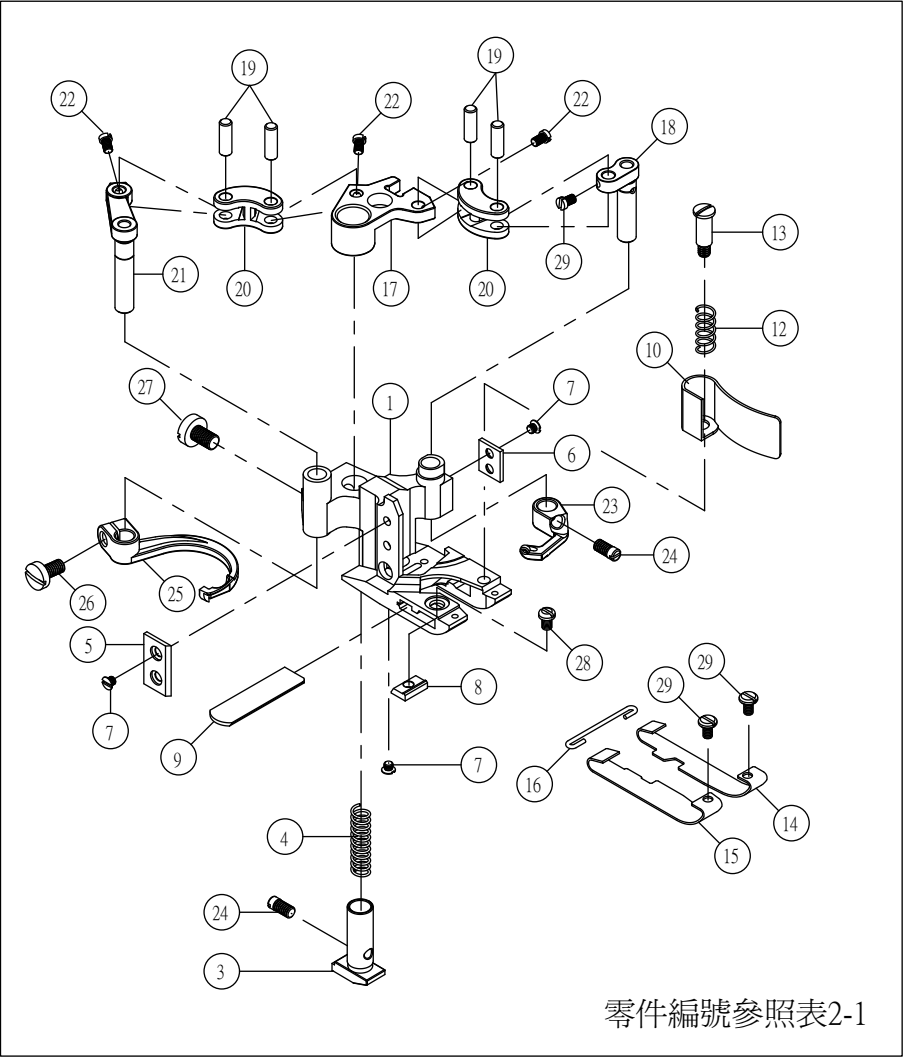
NT67-01 系列 壓腳組件(零件)一覽表
