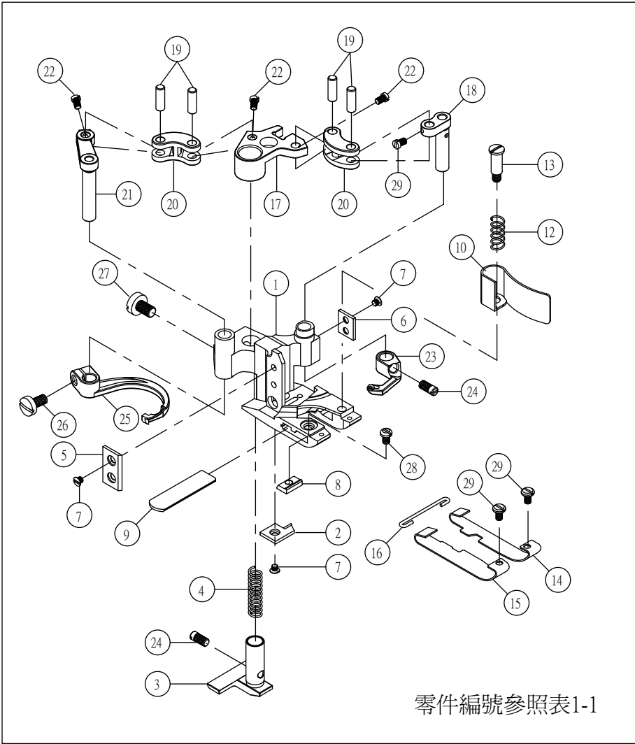
NT67-12 系列 壓腳組件(零件)一覽表
