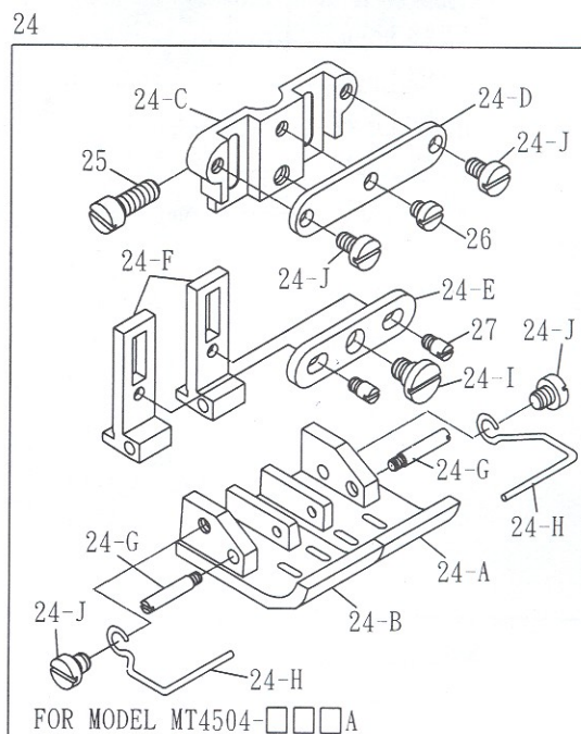
24-B PRESS FOOT
