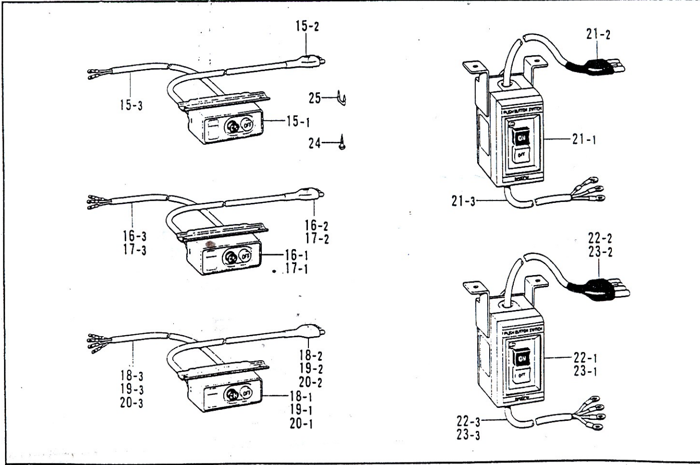
Q3. 電源スイッチ関係/Switch box mechanism/Schaltkasten/ Boîtier d'interrupteurs/Caja de interruptores
