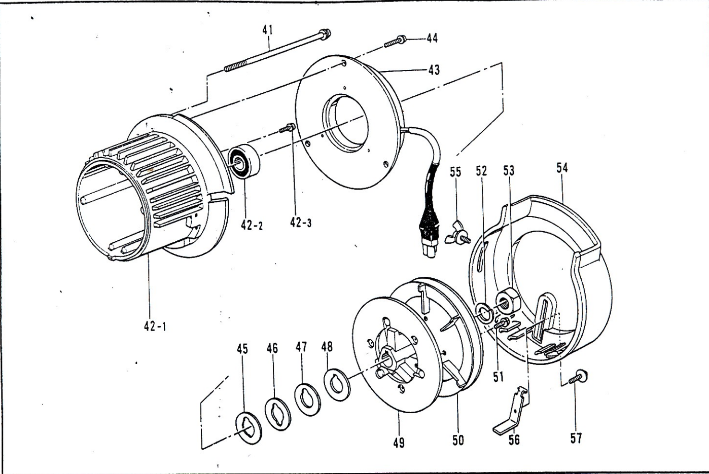
Q2. モーター関係(2)/Motor mechanism (2)/Motor (2)/ Mécanisme du moteur (2)/Mecanismo del motor (2)
