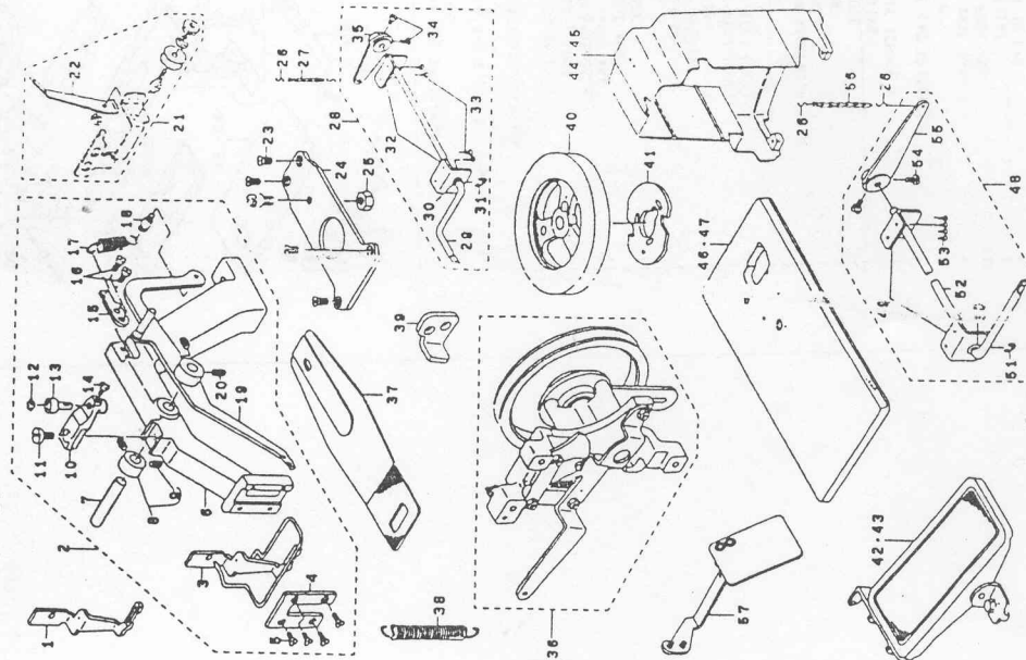
(15) LK-1854P-10 BELT LOOP ATTACHING MACHINE FOR P (21 STITCHES) P用21針バンド付けマシン
