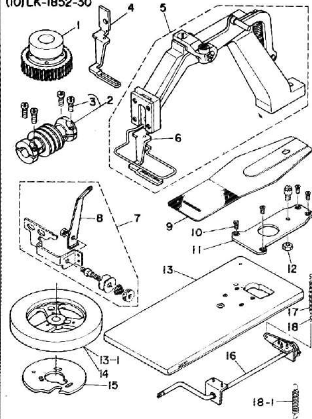
(10) LK-1852-30 BELT LOOP ATTACHING MACHINE (28 STITCHES) 28針バンドループ付けマシン
