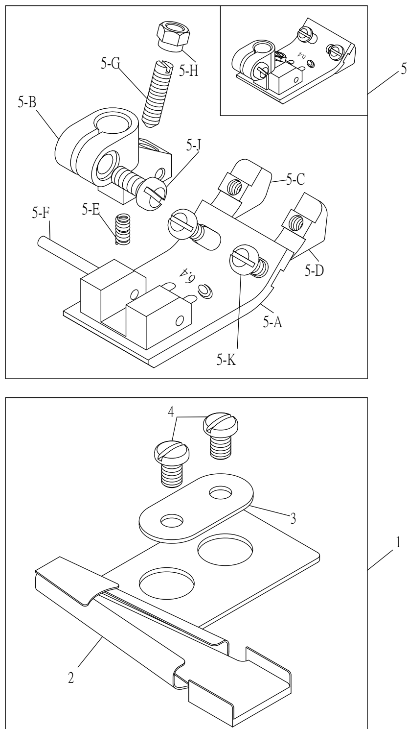
壓腳編號列表 Presser Foot
