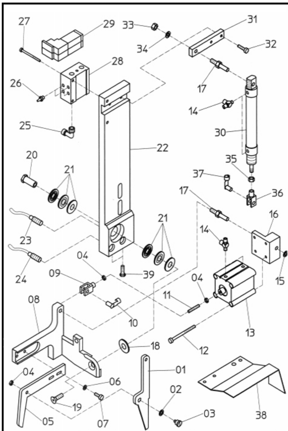
十二 Group12 拉链剪切装置 ZIP CUTTING ASSEMBLY 平缝自动开袋机 FLAP POCKET MACHINE
