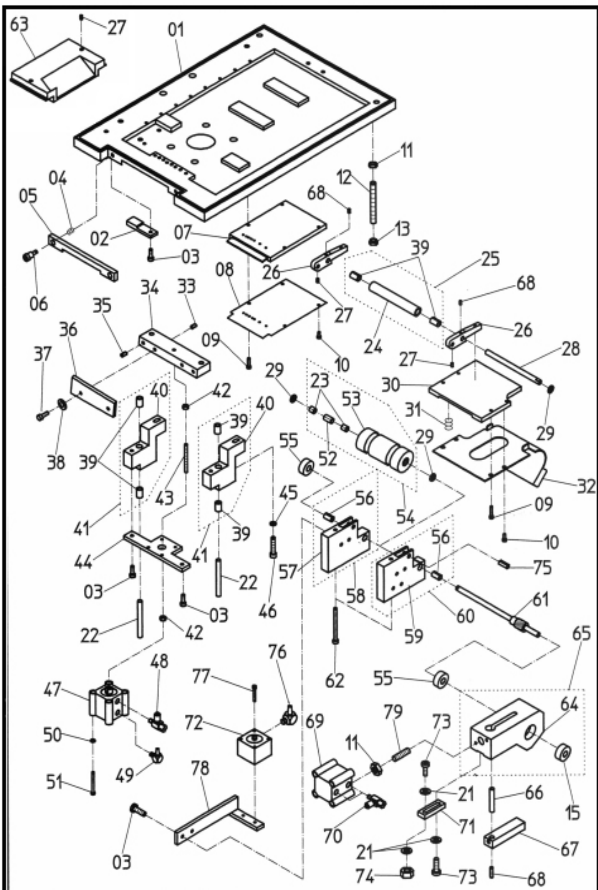
十三 里衬传送装置 平缝自动开袋机 Group 13 VACUUM WITH PELONFEED FLAP POCKET MACHINE
