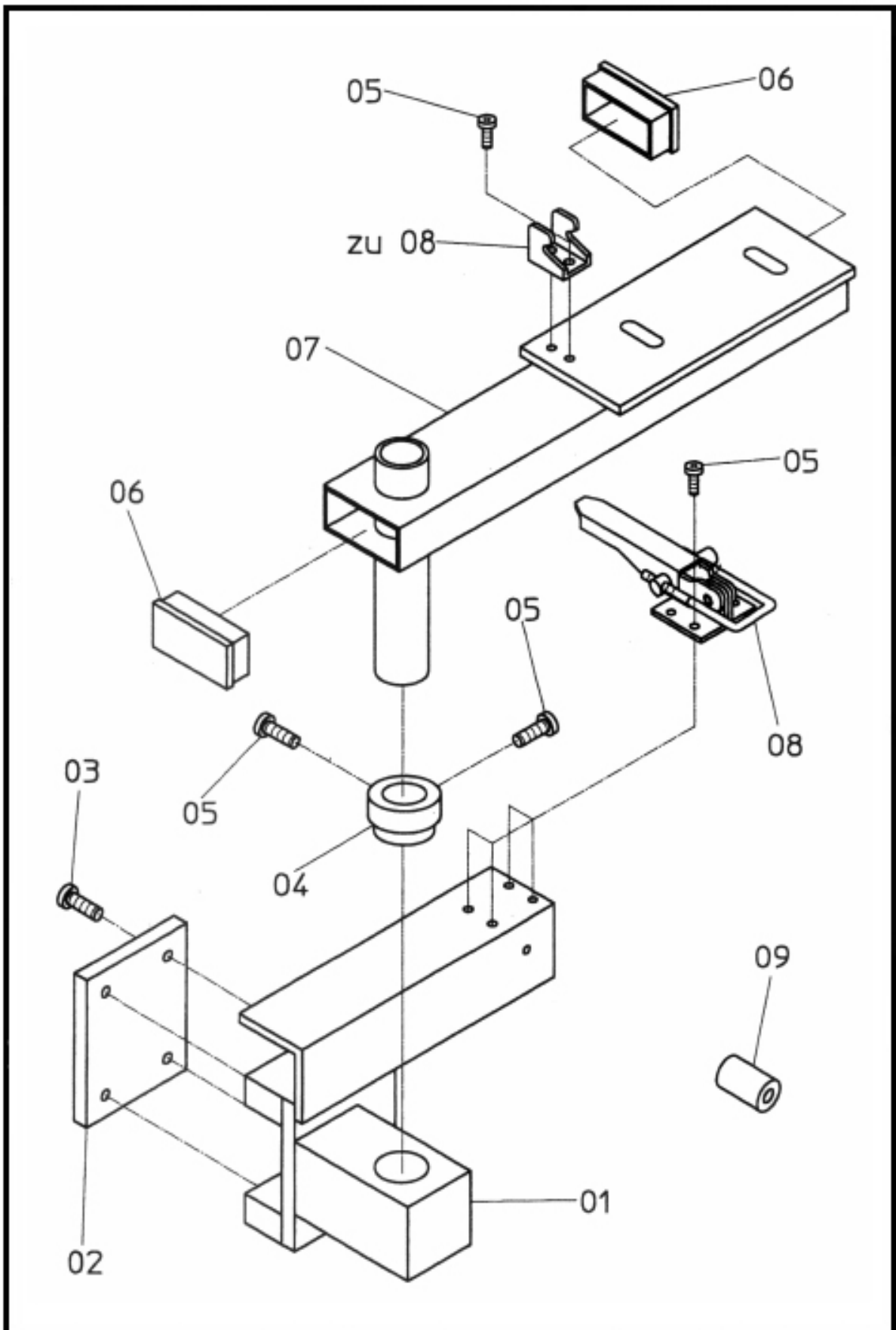
二十五 Group25 堆叠器连接臂 STACKER CONNECTOR ARM 平缝自动开袋机 FLAP POCKET MACHINE
