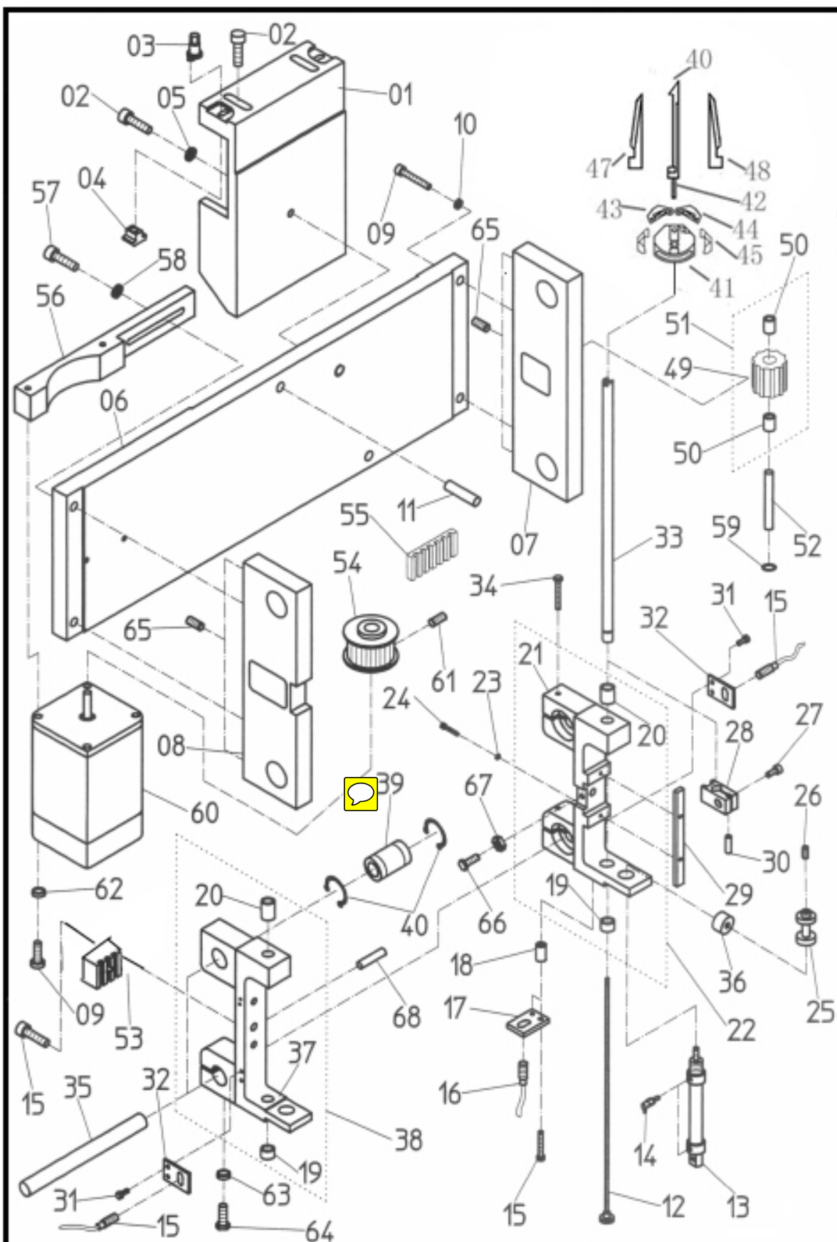
七 Group 7 角刀机构 (一) TAB KNIFE ASSEMBLY 平缝自动开袋机 FLAP POCKET MACHINE
