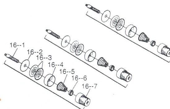
五线夹线器组件图示
