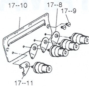
四线夹线组件图示
