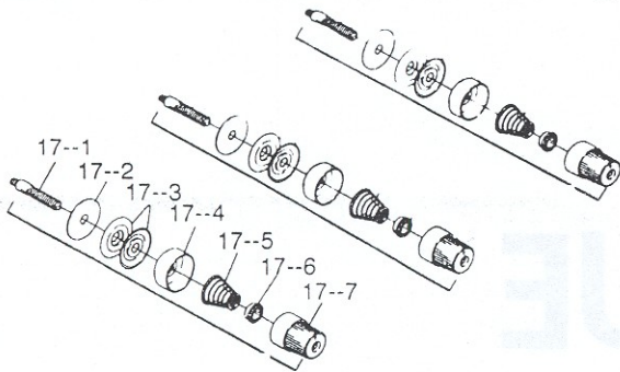
三线夹线组件图示
