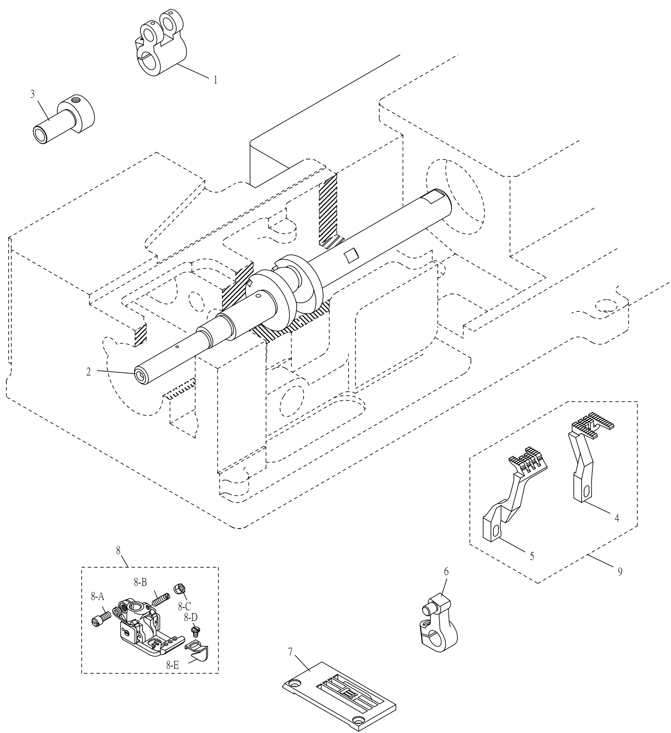
7. 針板 Needle Plate
