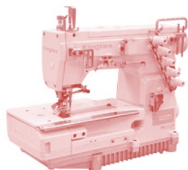
FT7000-0-356M General Plain Seaming 一般車(平)縫
