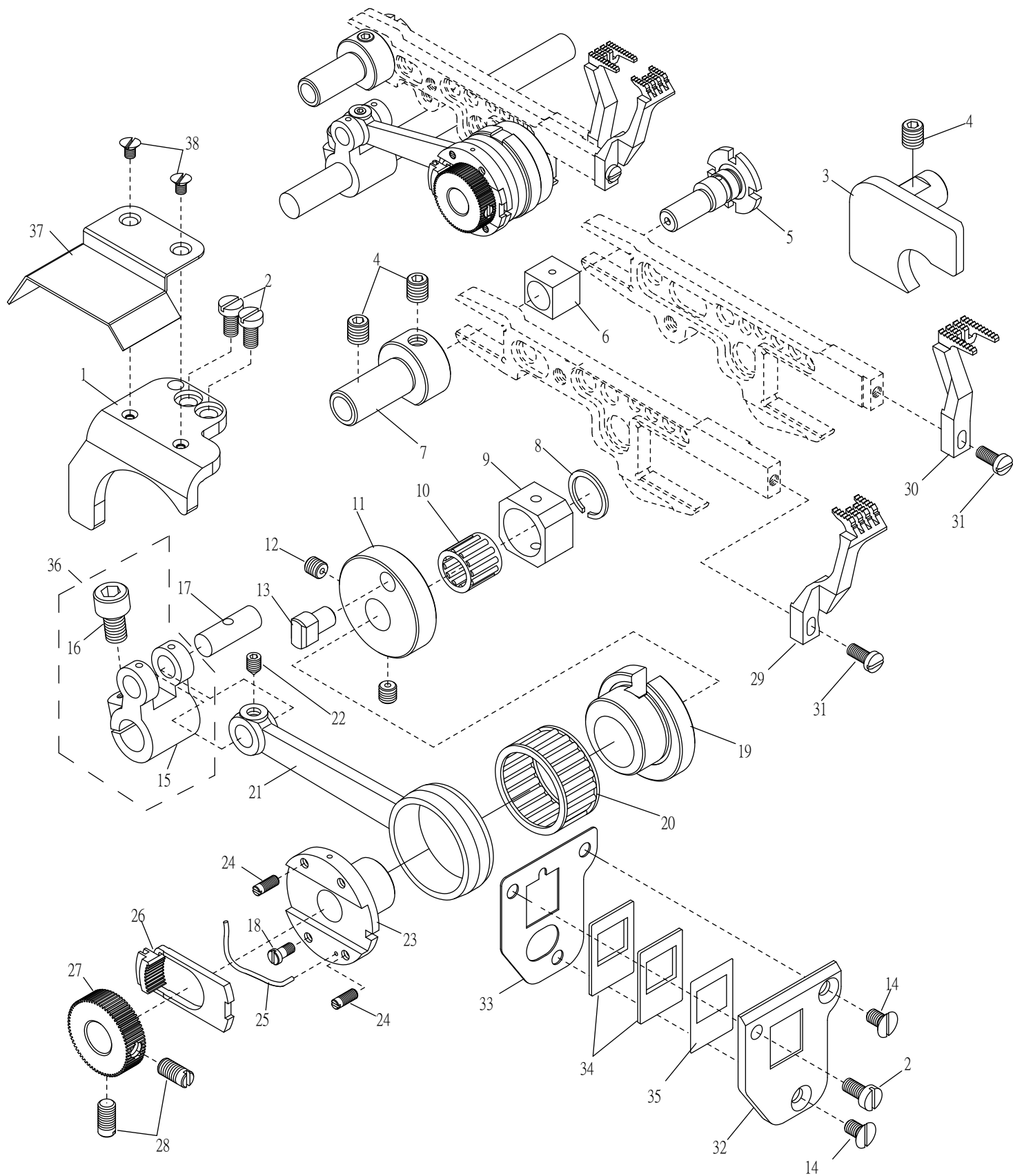
30. 主送齒編號列表 Main Feed Dog
