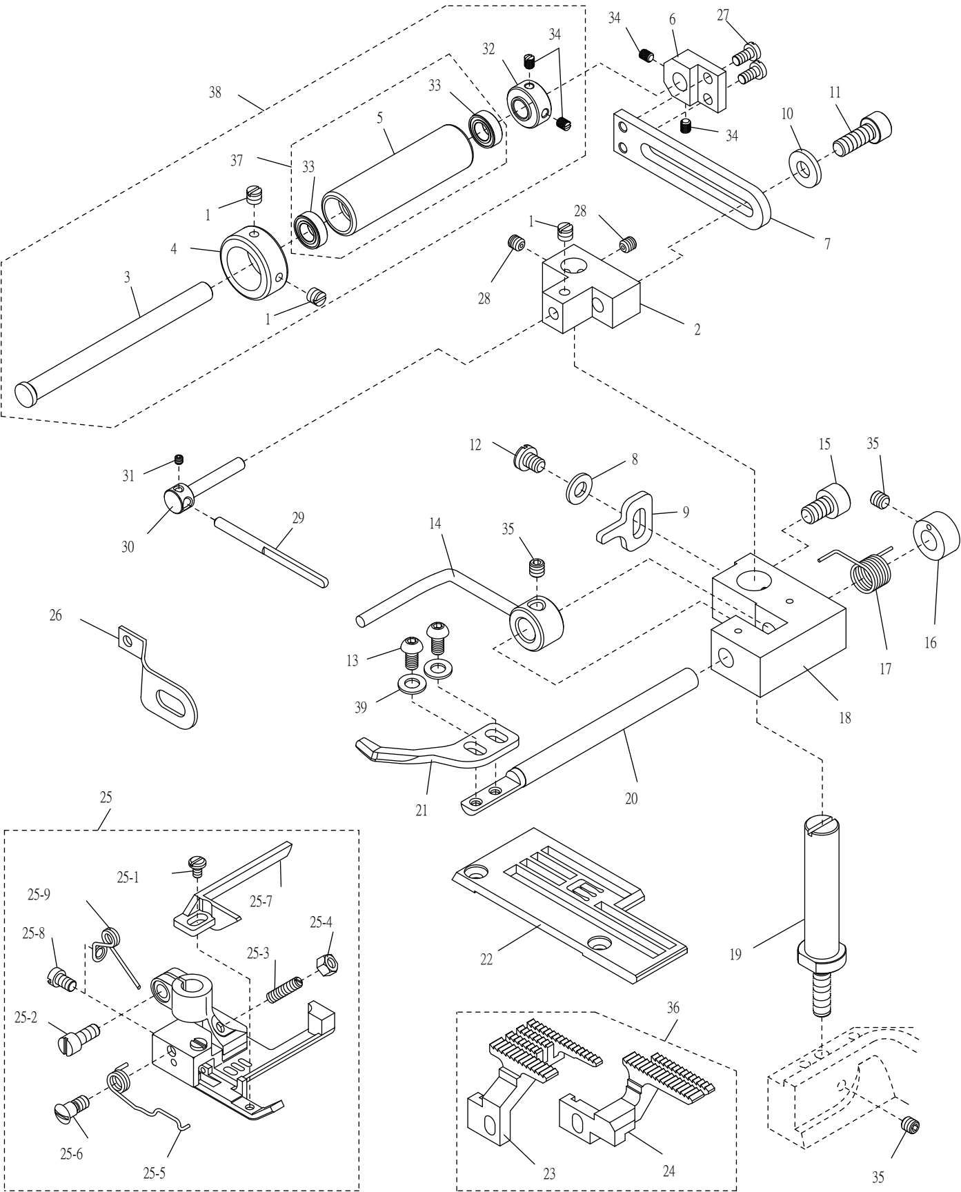
25. 壓腳編號列表 Press Foot
