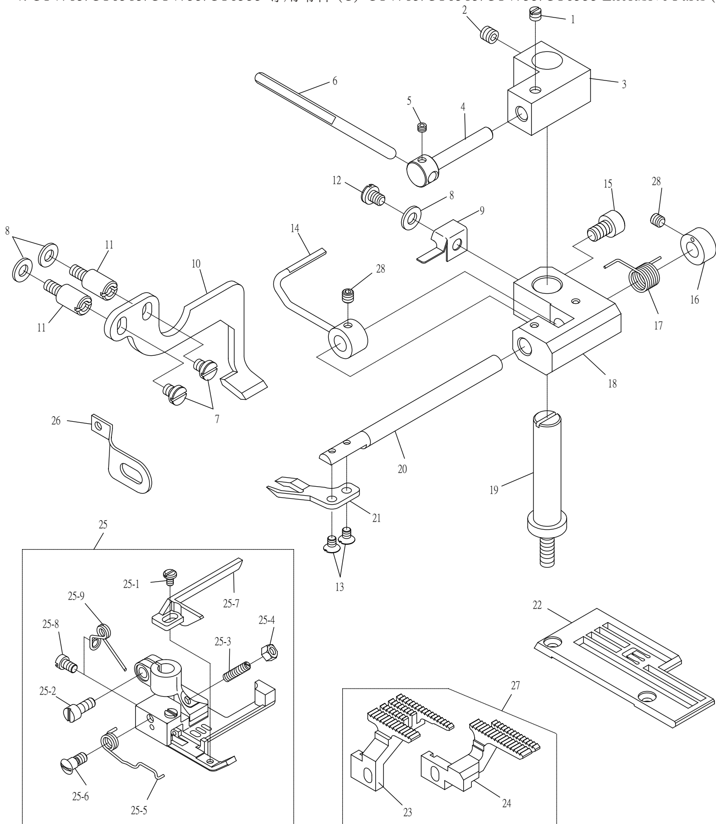
25. 壓腳編號列表 Press Foot
