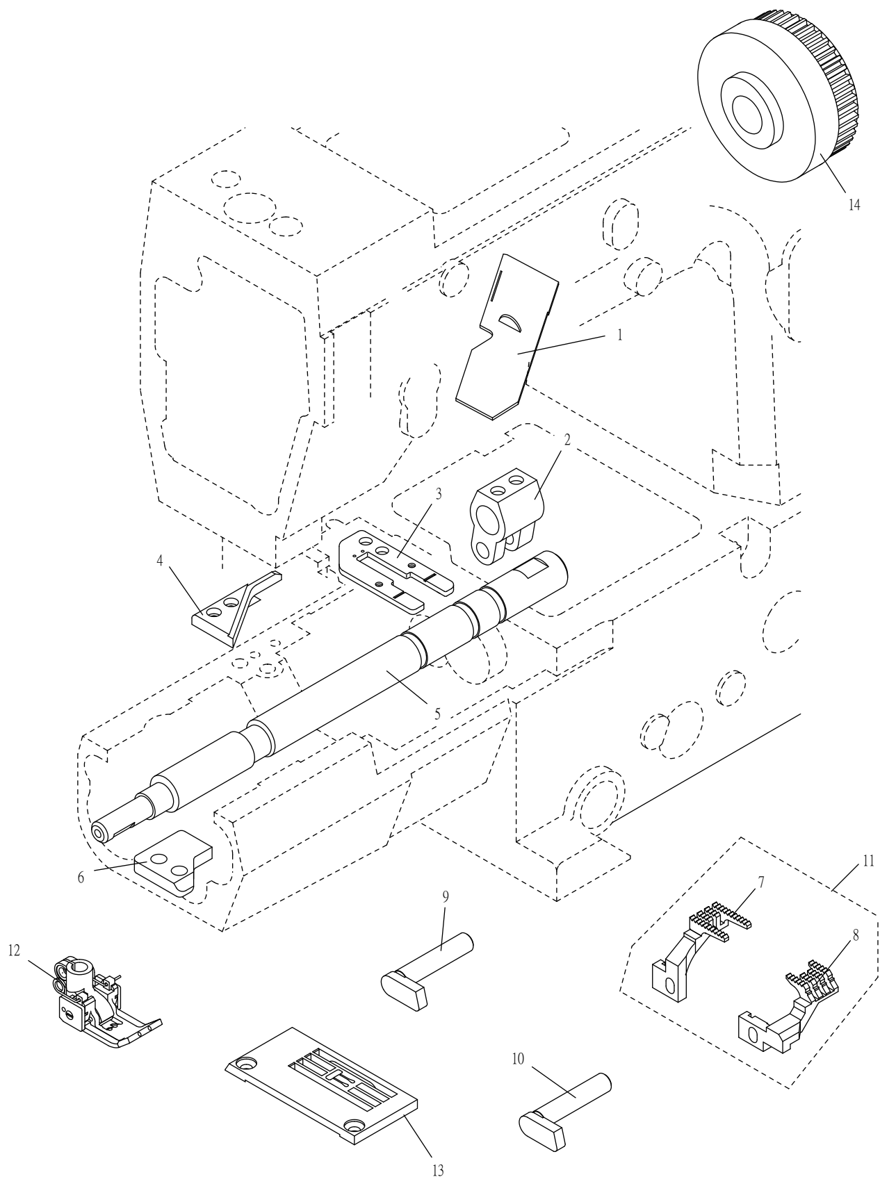
12. 壓腳組 Presser Foot
