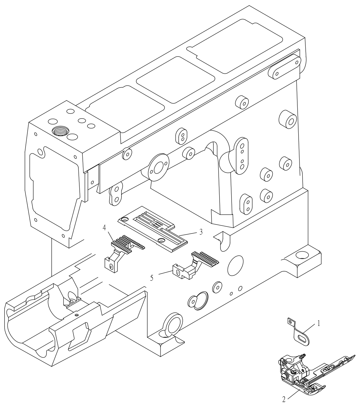
2. 壓腳編號列表 Press Foot
