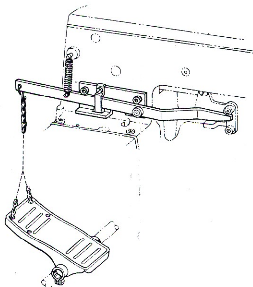
メカ・ツーペダルセット Mechanical two-pedal set S03655-001
