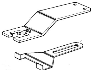
ラベル付アタッチメント組 Label attachment S03692-001
