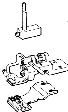
シャンクアタッチメント組 Shank button attachment 142570-201
