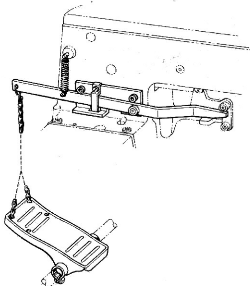
メカ・ツープダルセット Mechanical two-pedal set S03655-002
