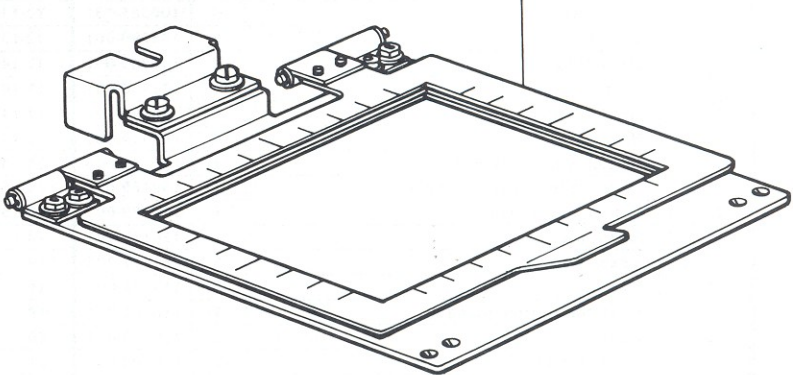
Hoop (D) Assembly 157274-001
