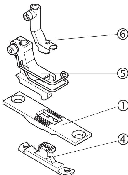
E265
