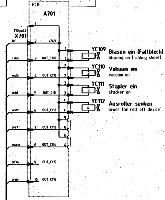
Leiterplatte k 9850 001070
