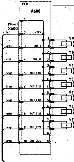
Leiterplatte k 9850 001060
