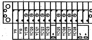
Leiterplatte k 9850 001070
