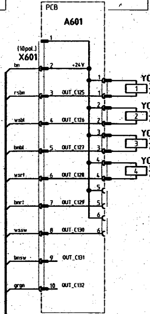
Leiterplatte k 9850 001070
