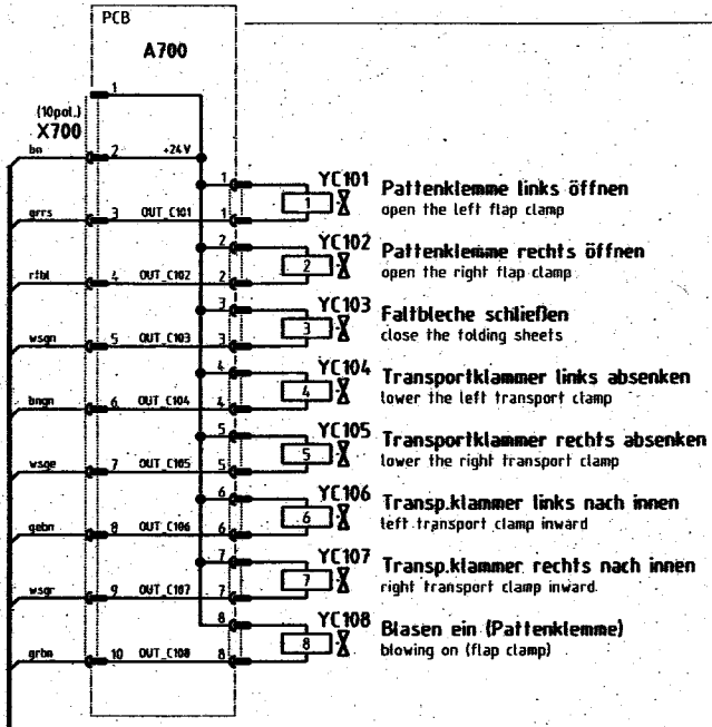
Leiterplatte k 9850 001060
