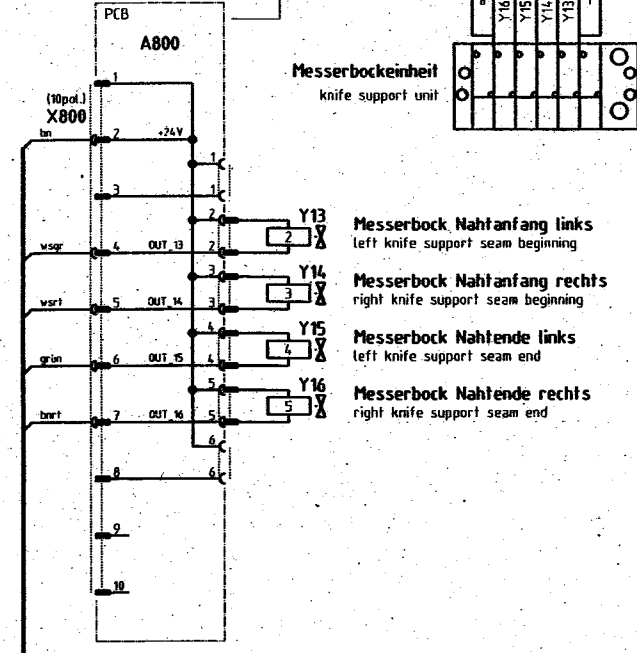
Leiterplatte k 9850 001070
