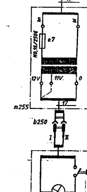
⑪ Bei 230V u. 240V Primärspannung Lampe an 11V anschließen When prim. Voltage 230V or 240V connect lamp to 11V
