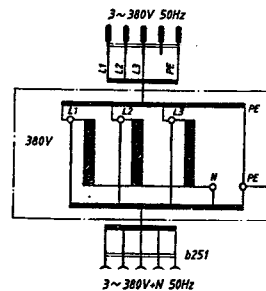
④ Spartransformator zur Anpassung einer für 3~380V-N ausgelegten Maschine an eine Netzspannung von 3~380V ohne Mittelpunktsleiter (N)
