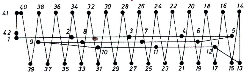
Nahtbild der DÜRKOPP 570-104205 Seam pattern of DÜRKOPP 570-114211/E59;/E159
