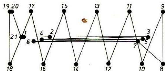
Nahtbild der DÜRKOPP 570-124206/E551 Seam pattern of DÜRKOPP 570-124206/E551 -134206/
